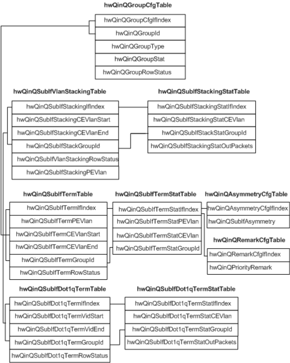
图 103-2 子接口 QinQ 配置表的表间关系图
