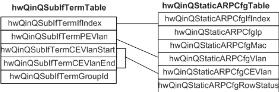
图 103-4 子接口终结配置表与静态 ARP 配置表的关系
