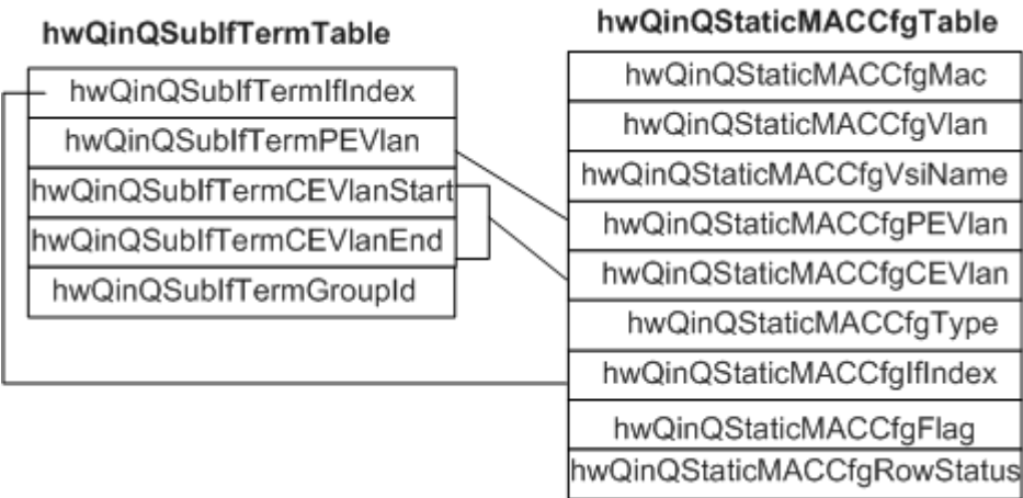
图 103-3 子接口终结配置表与静态 MAC 配置表的关系
